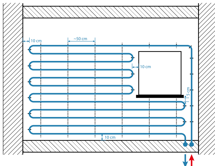
Slika 34. Razmaci kod postavljanja sistema za grijanje zida.
