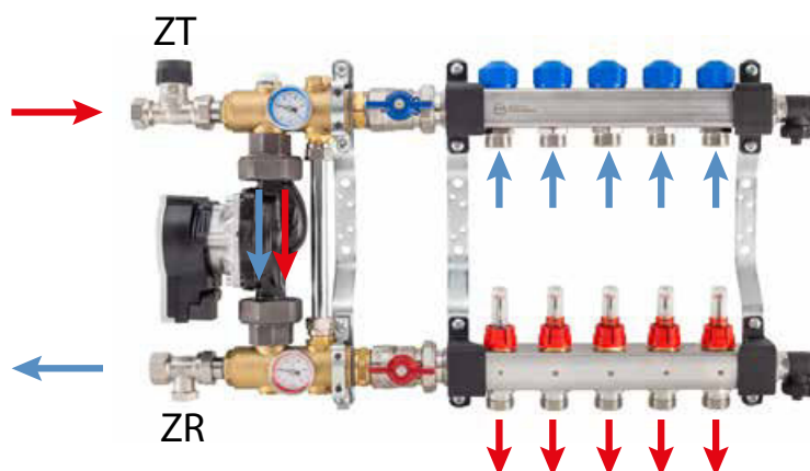
Slika 57. Razdjelnik opremljen USFP-om sa sistemom jedinice za miješanje – smjerovi protoka.
