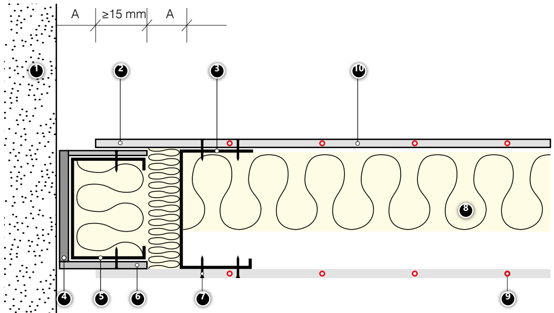
Slika 41. Klizni spojevi sa zidom
