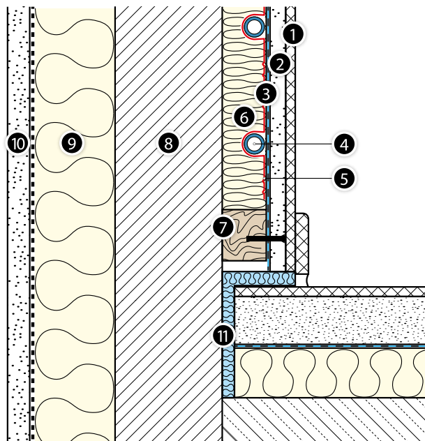
Slika 36. KAN-therm TBS sistem za grijanje zidova
