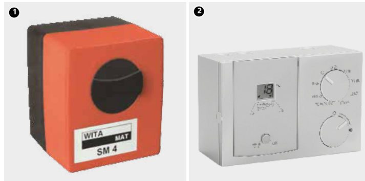
Slika 52. Regulacijski elementi KAN-therm centralnog sistema mješanja (SM4 aktuator (1) regulator vremena(2))
